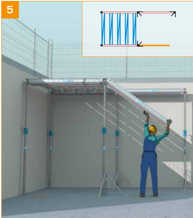
- Anbringen eines Hauptträgers auf einer mit Dreibeinen stabilisierten Schalungsstütze (ST).
